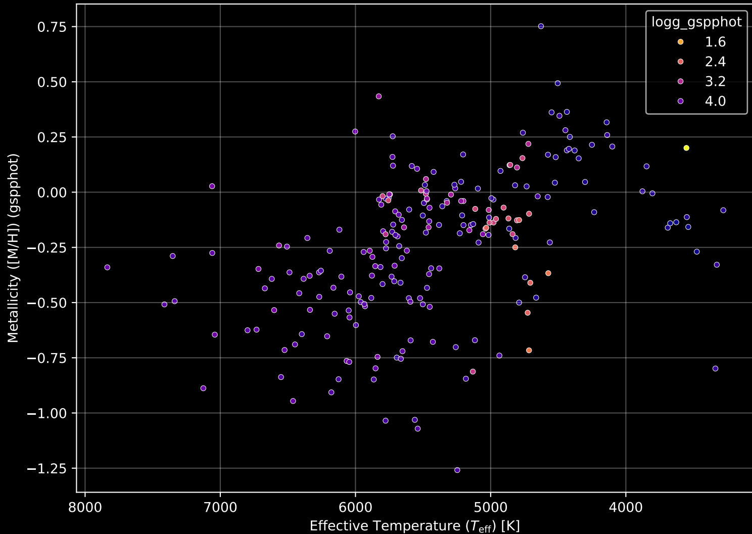
APOGEE DR17 Field: [185-42_MGA] Stellar Population Parameters (n= 223)
